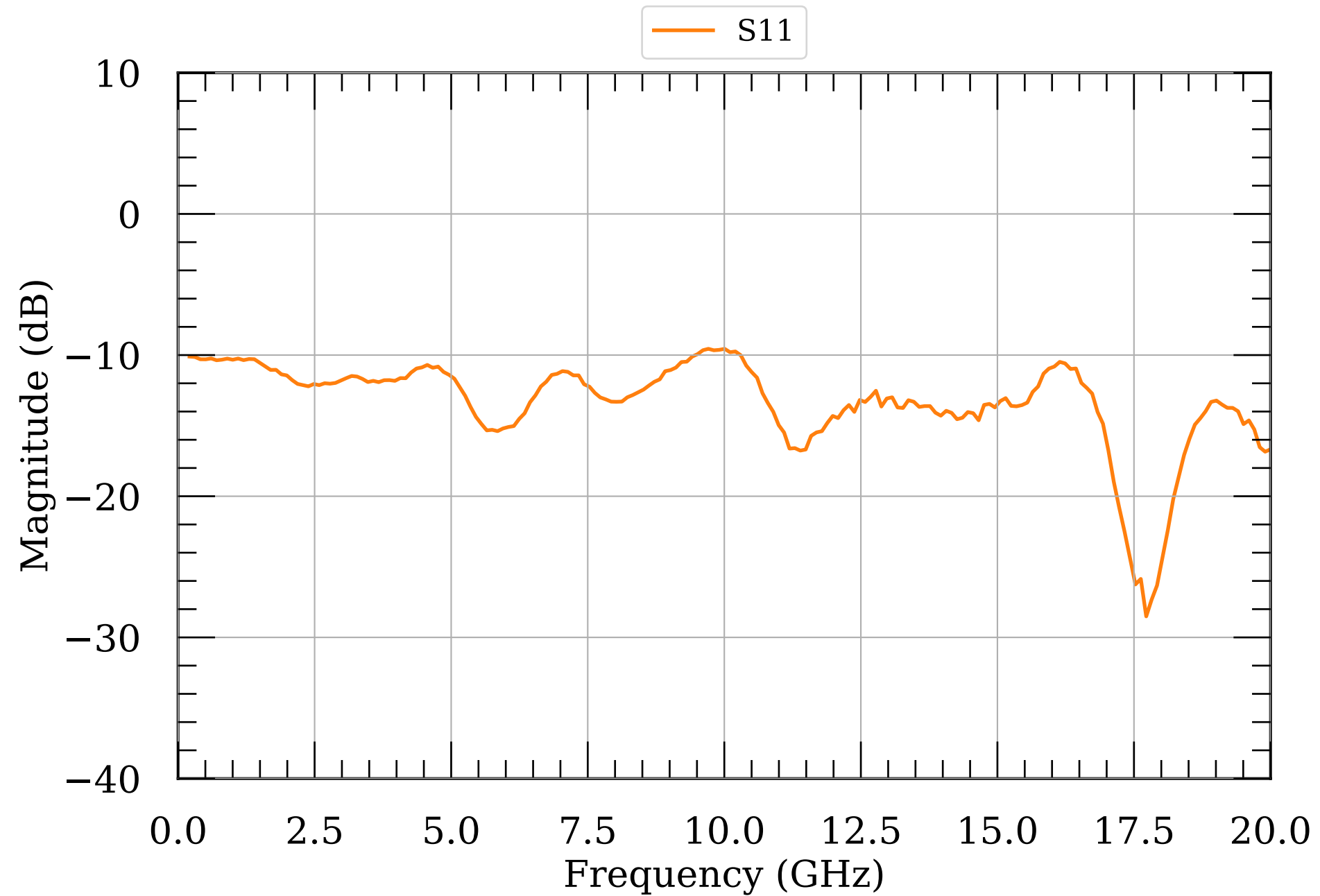
LNA S-params module068v2
